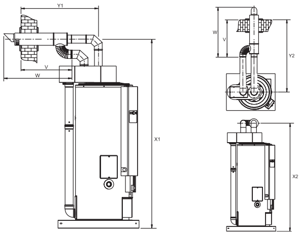
Muurafvoer concentrisch
