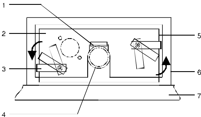
Figure 7 - Montage du portillon
